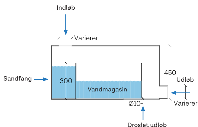
Snit teknikkasse - set forfra
