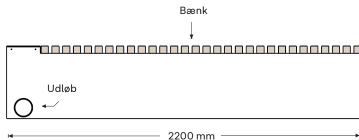
Snit - set fra siden
