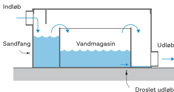
Snit teknikkasse - set forfra
