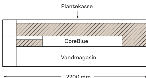
Snit - set fra siden
