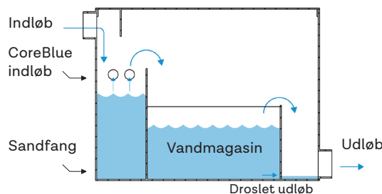
Snit teknikkasse - set forfra
