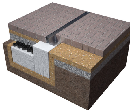
CoreBlue+™ D34 med integrert avløp og rist
