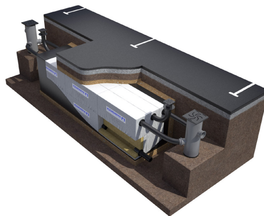
CoreBlue+™ BD med integrert rørføring til brønn
