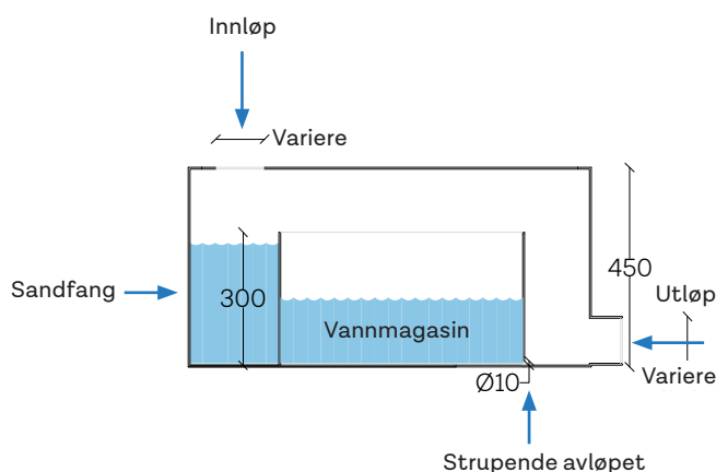
Utsnitt av teknisk boks - sett forfra
