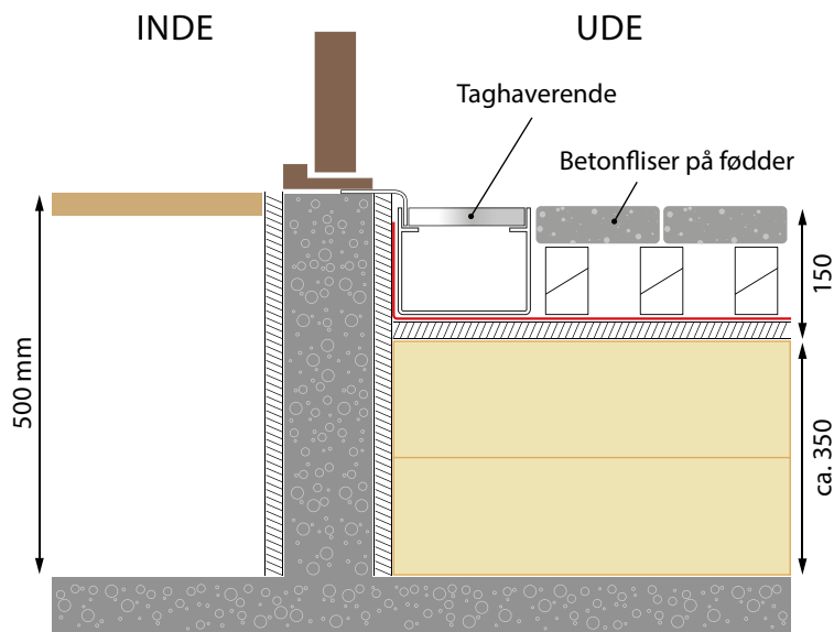
Figur 1. Varmt tag med høj gulvopbygning og terrassegulv med betonfliser. Højdeforskel ved dør maks. 25 mm.
