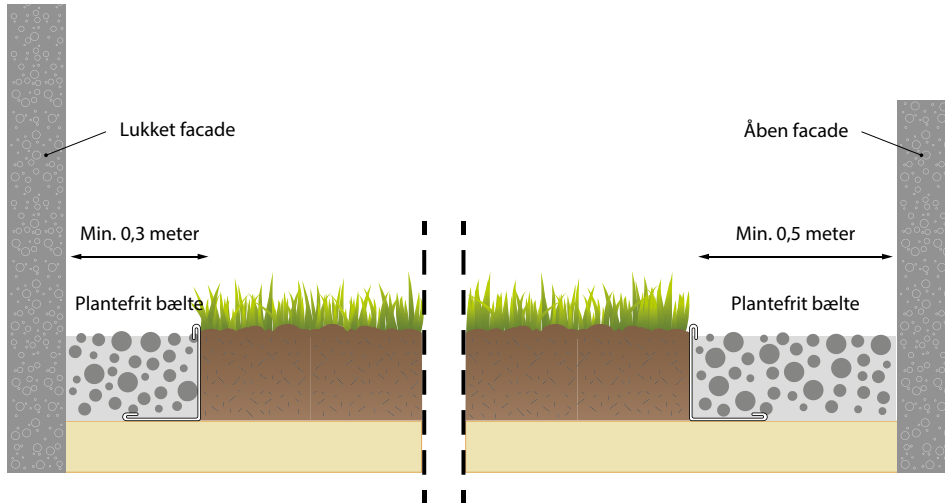
Figur 1. Brandbælter.
