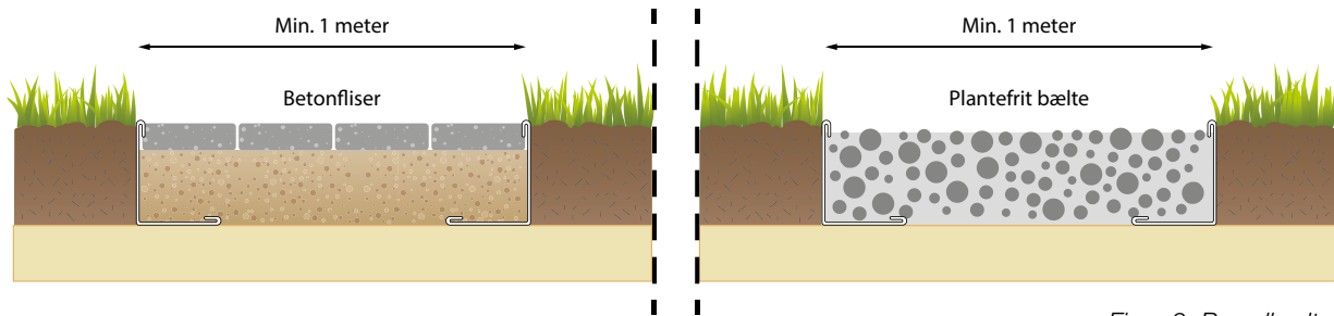
Figur 2. Brandbælter.
