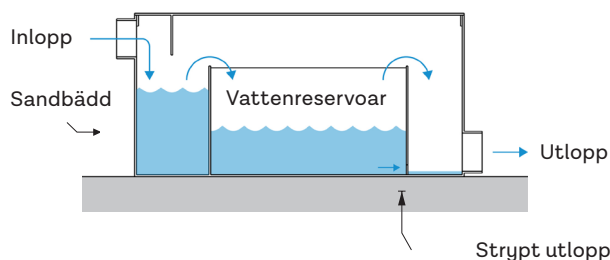
Delad teknisklåda - sett framifrån
