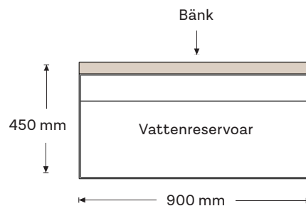
Delad - sett framifrån
